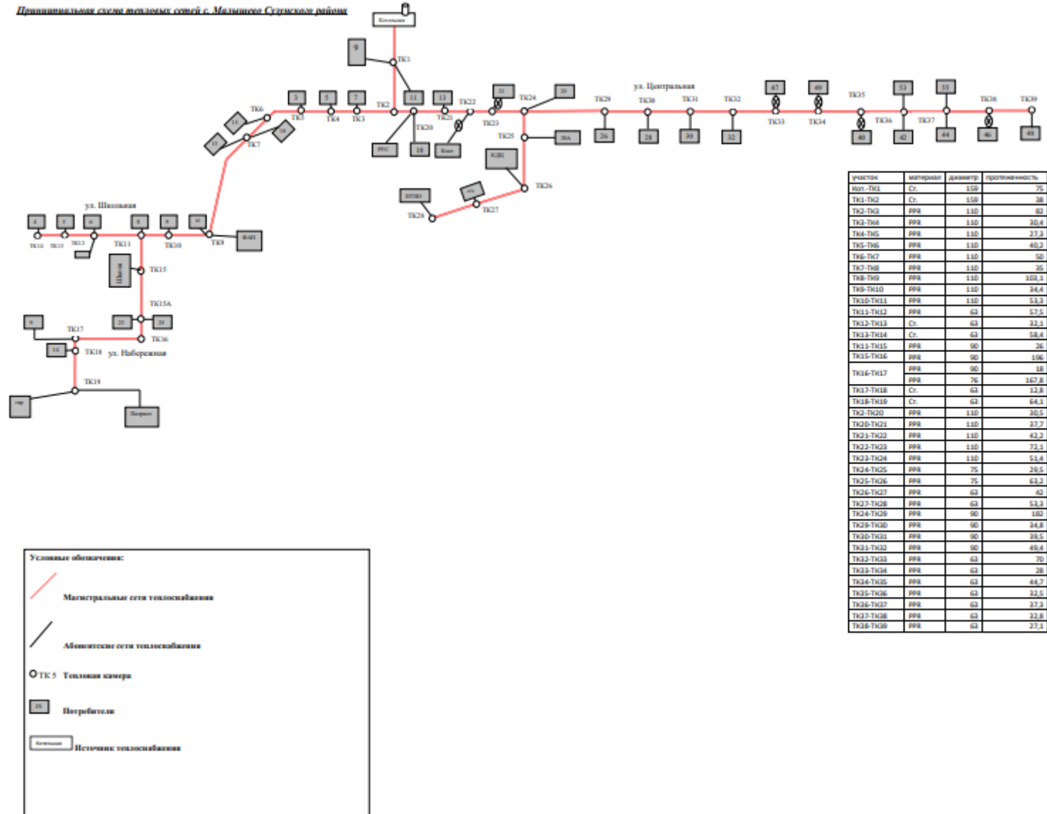
Рисунок 2. Схема тепловых сетей от котельной по ул. Центральная.
