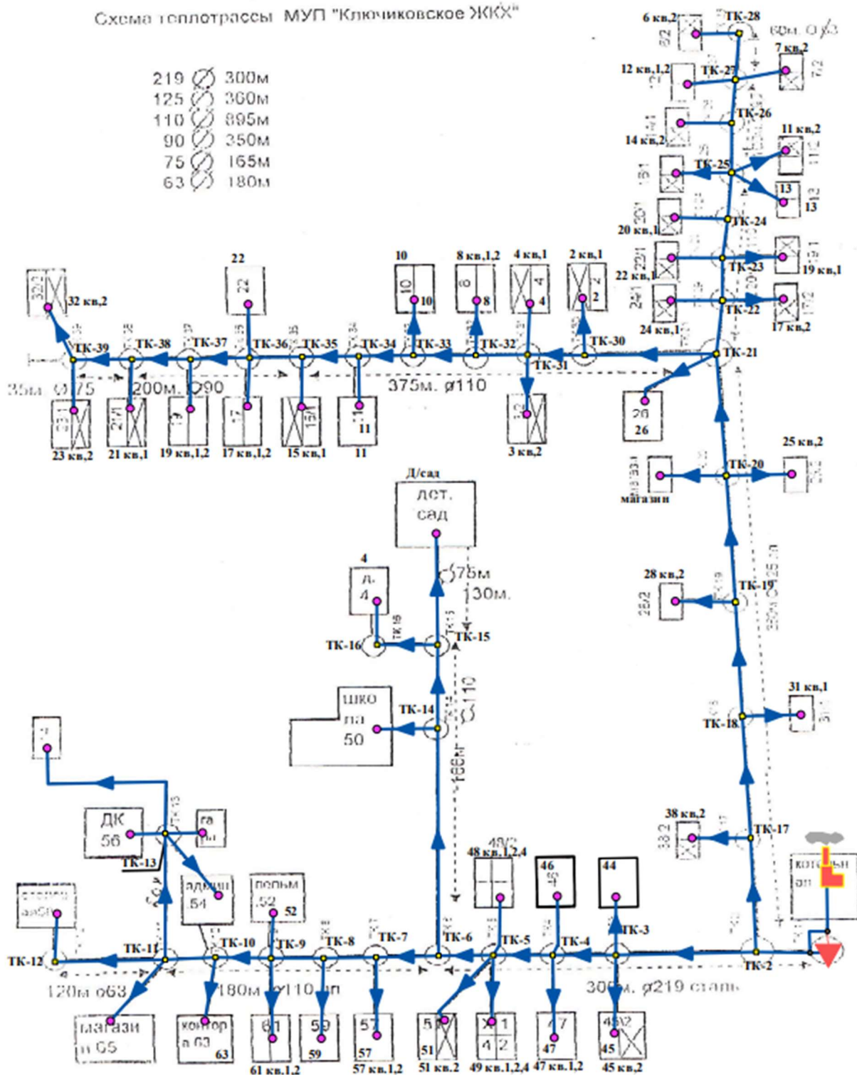
Рисунок 2. Схема тепловых сетей от котельной по ул. Кирова.
