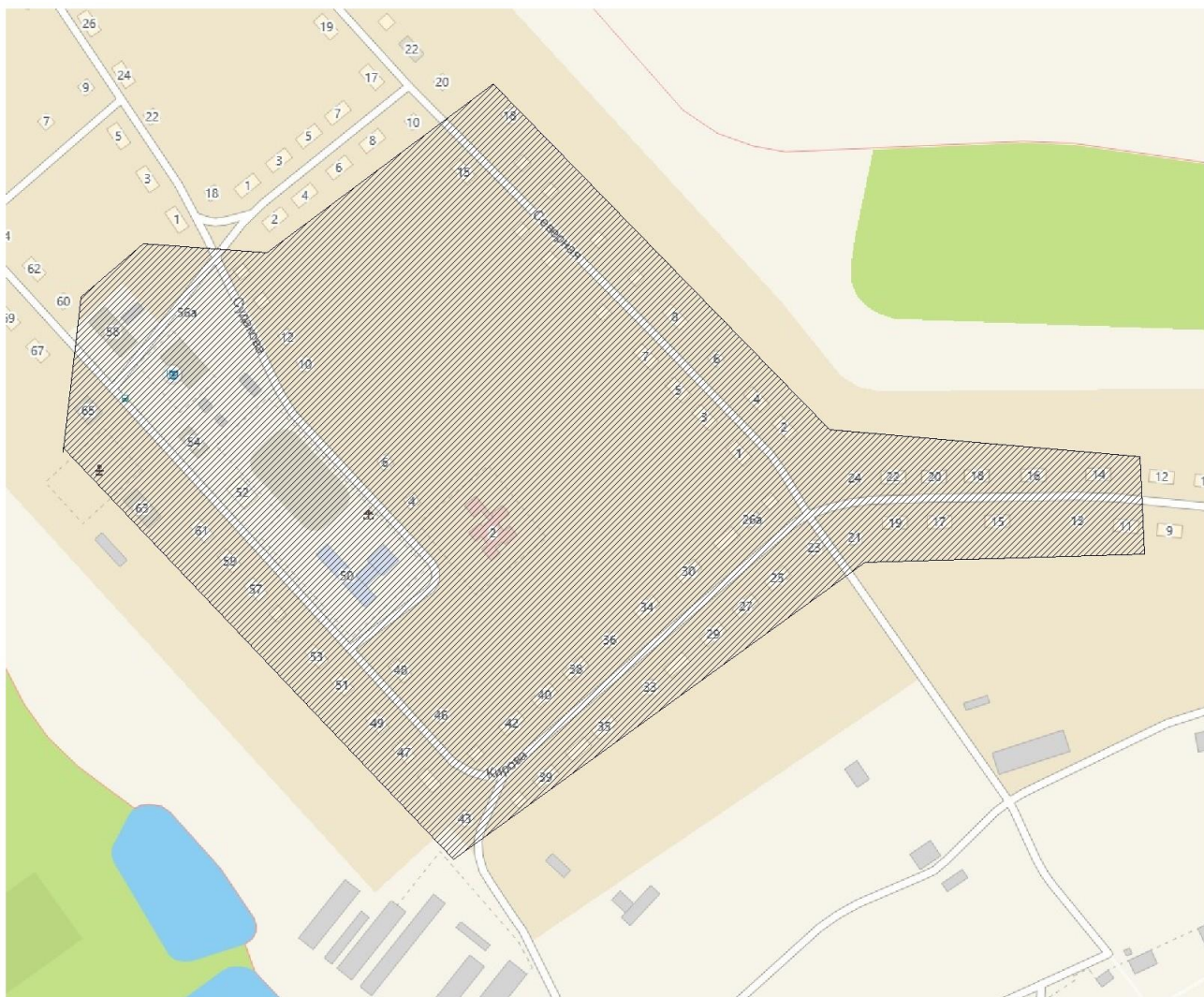
Рисунок 3. Зона действия котельной МУП «Бобровское ЖКХ» по ул. Кирова.
