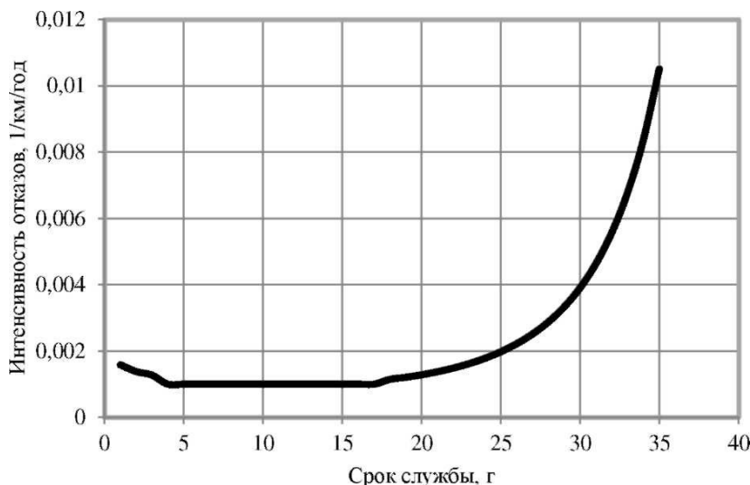
Рисунок 3. Интенсивность отказов в зависимости от срока эксплуатации участка тепловой сети
