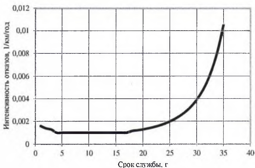
Рисунок 4. Интенсивность отказов в зависимости от срока эксплуатации участка тепловой сети
