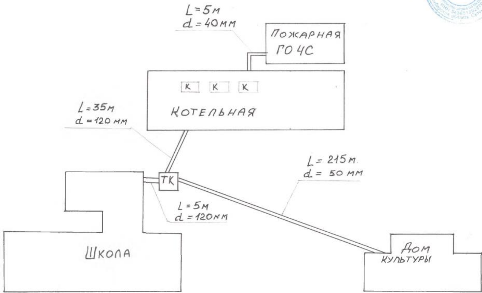
Рисунок 2. Схема тепловых сетей от котельной по Центральный переулок, 16.
