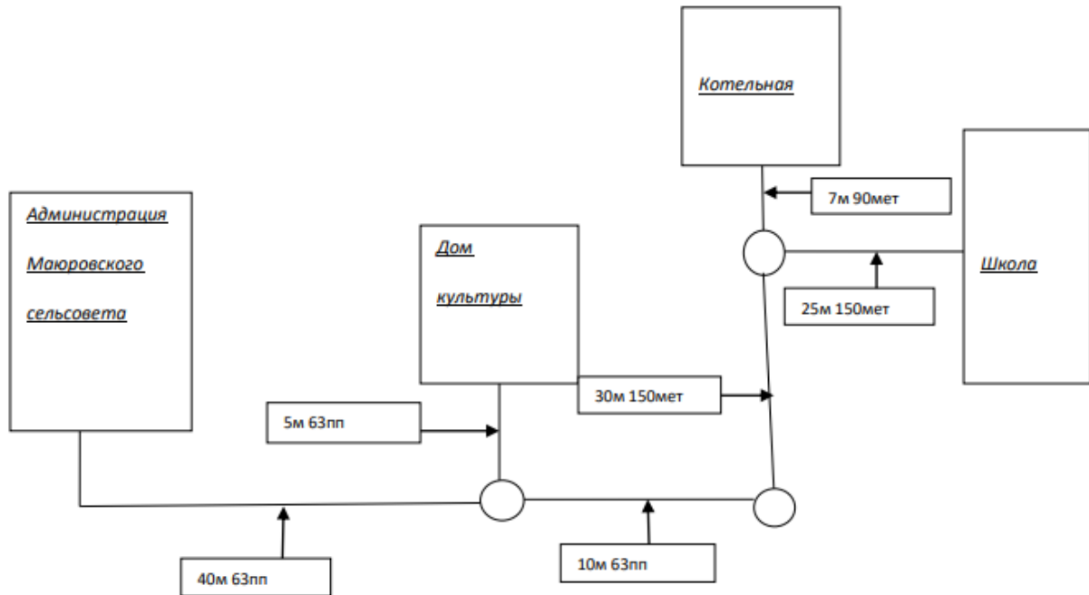
Рисунок 2. Схема тепловых сетей от котельной по ул. Центральная, 15а
